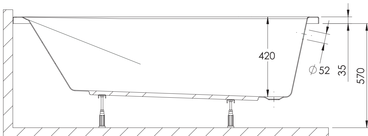
ŘEZ A-A
